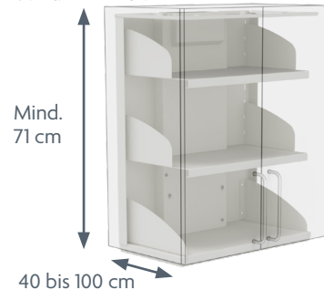
Abmessungen des höhenverstellbaren Systems
