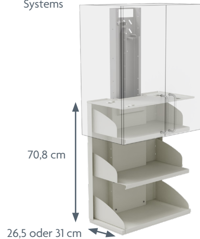
Abmessungen des höhenverstellbaren Systems
